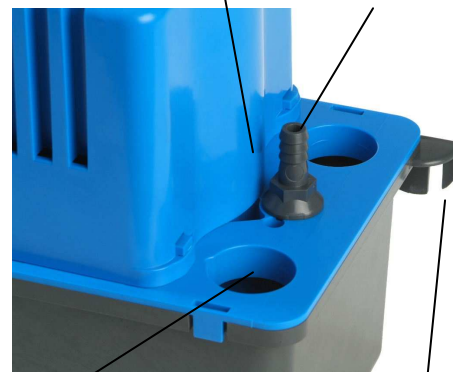
Integriertes Rückschlagventil
